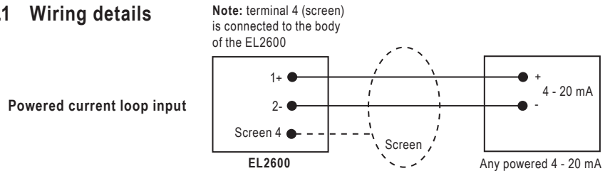
Fig. 2 Wiring details
