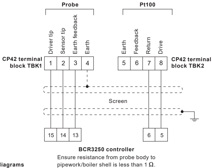
Fig. 4 Wiring diagrams
