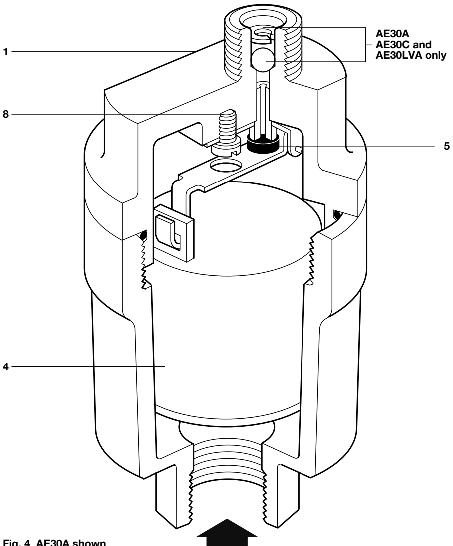
Fig. 4 AE30A shown
