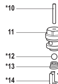
Explosionszeichnung der Position 11
