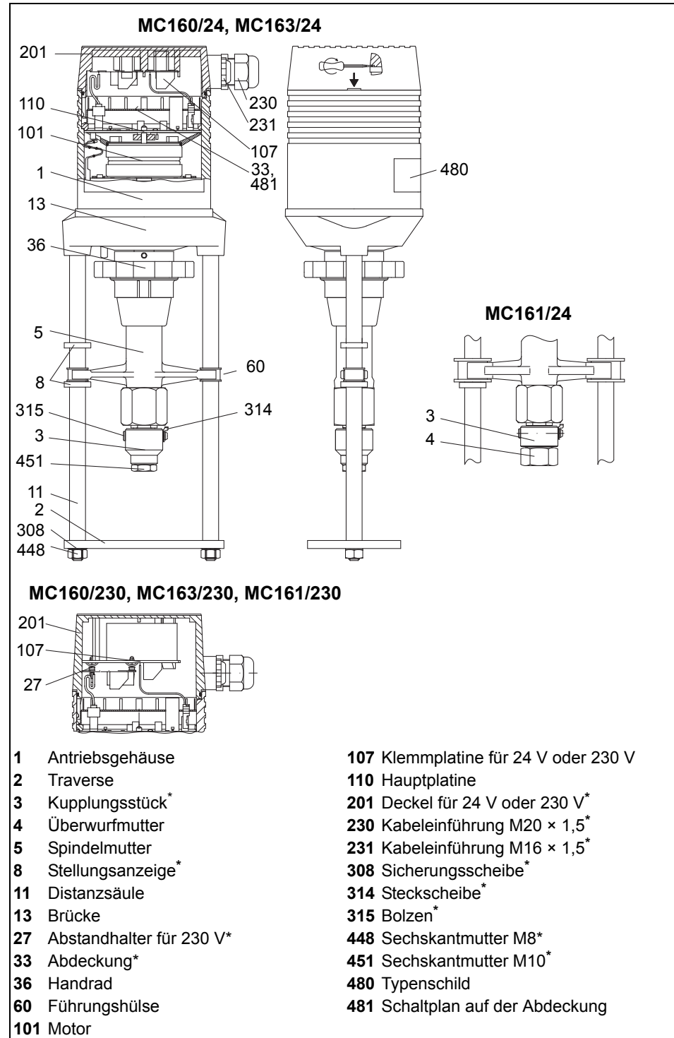
Bild 1 Bauteilbezeichnungen
