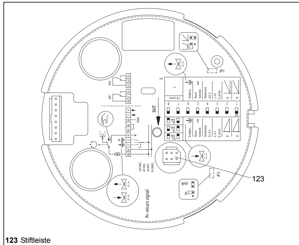
Bild 12 Stiftleiste für Wegschalterplatte auf der Hauptplatte
