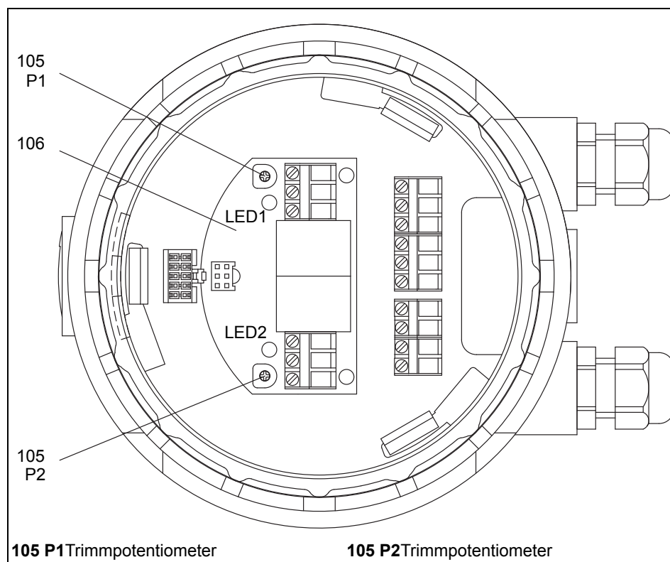
Bild 18 Wegschalterplatine im Deckel
