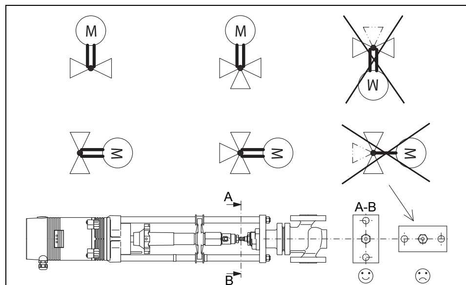
Bild 5 Einbaulagen von Hubantrieb und Ventil
