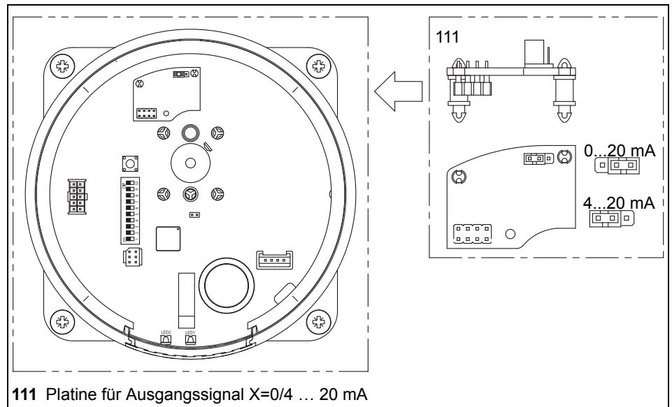
Bild 2 Platine für mA-Ausgangssignal auf der Hauptplatine
