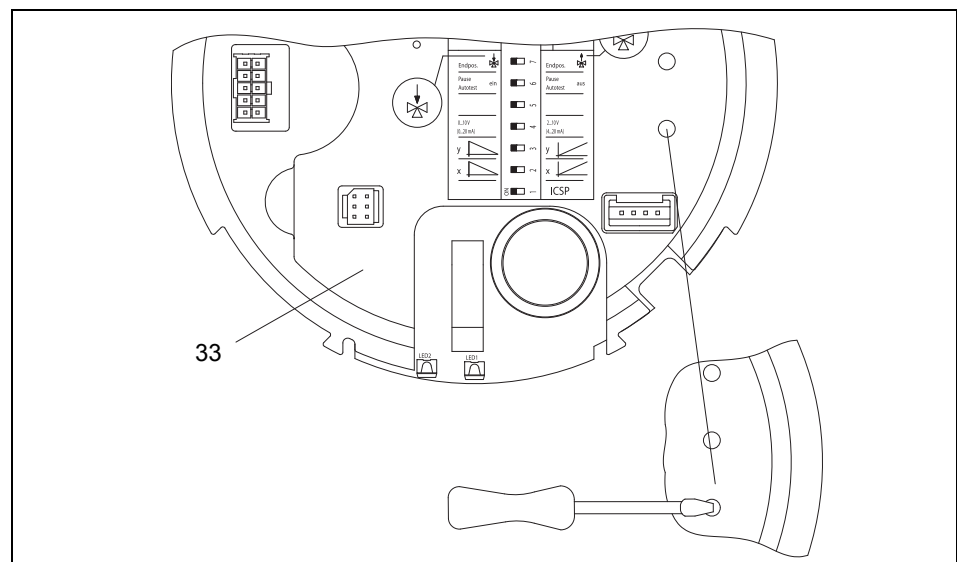
Bild 10 Platinenabdeckung im Antriebsgehäuse abnehmen
