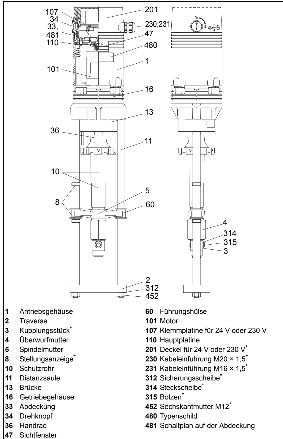
Bild 1 Bauteilbezeichnungen
