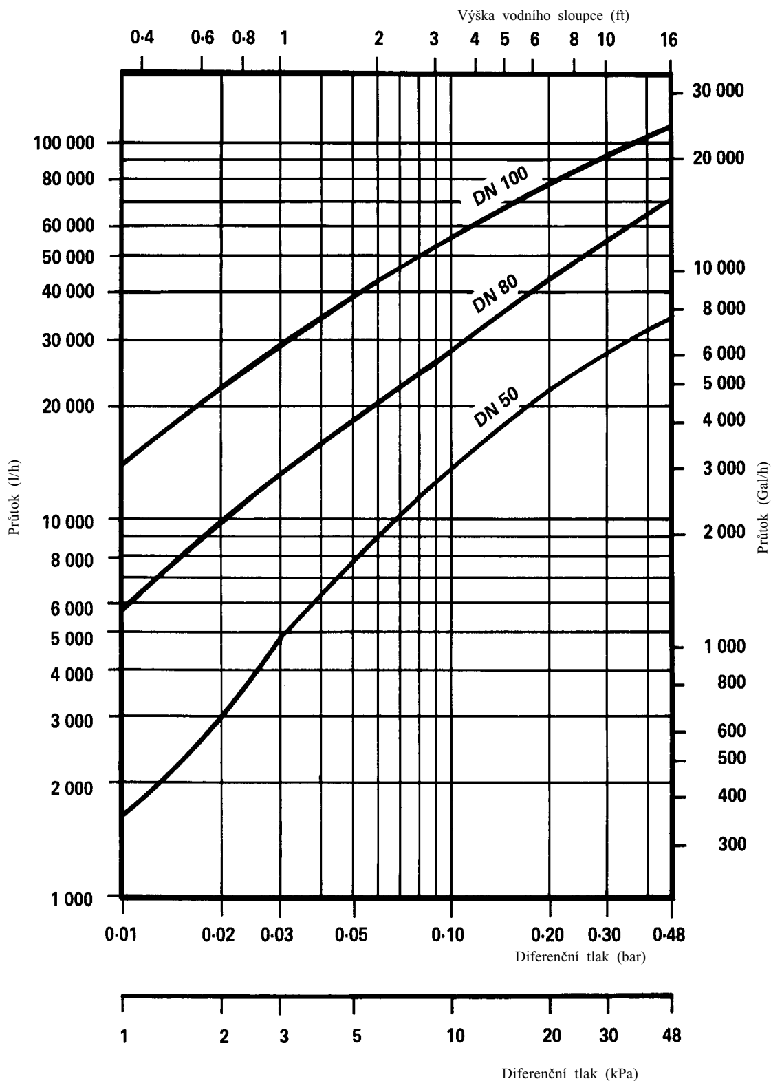
Graf dimenzování ventilu pro vodu
