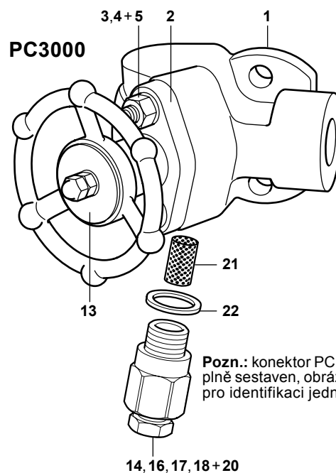
Vnitřní části pístového ventilu
