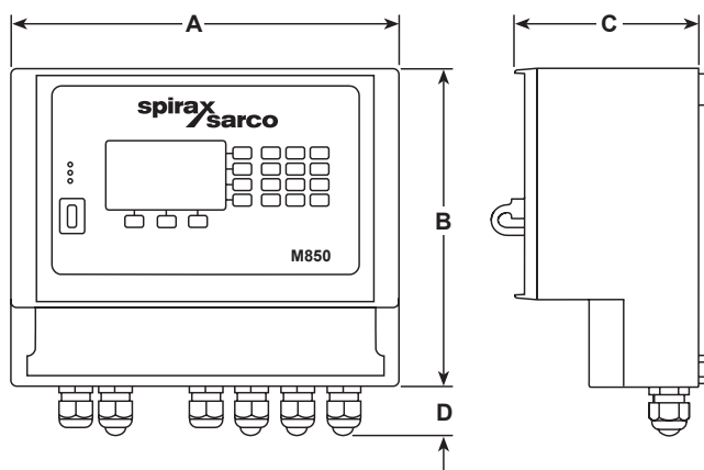
M850-W-x (montáž na stěnu)
