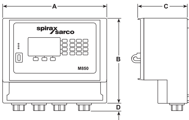
M850-W-x-UL (montáž na stěnu)
