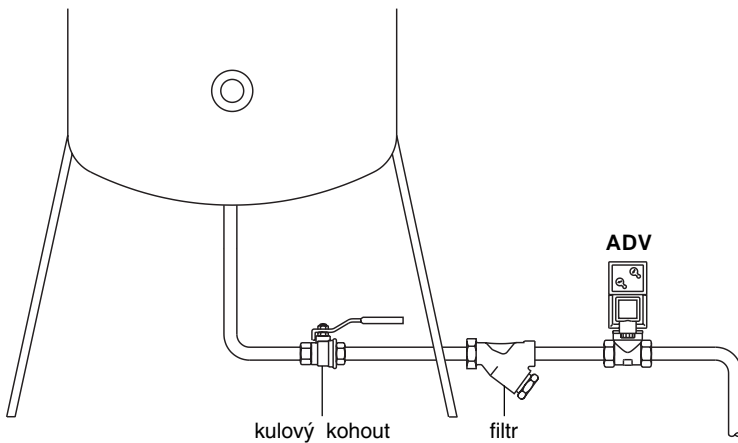
Obrázek 1: Odvodnění zásobníku tlakového vzduchu (nebo rozměrného filtru)
