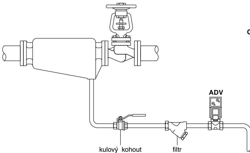
Obrázek 3: Odvodnění separátoru na hlavním potrubí tlakového vzduchu
