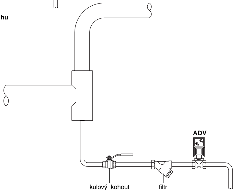
Obrázek 2: Odvodnění rozvodu tlakového vzduchu
