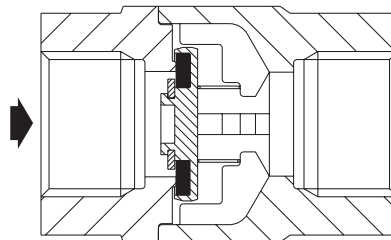
Obr. 2 Verze s měkkým těsněním (pouze závitové verze)
