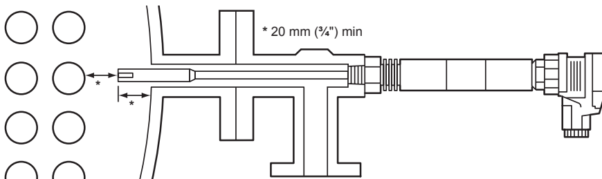
Obr. 3 Typická instalace sondy do "T" kusu (kolene) - pouze závit 3/8" BSP
