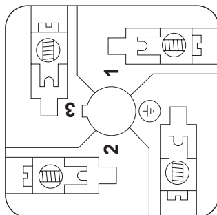
Obr. 9 Pohled na blok svorek konektoru sondy
