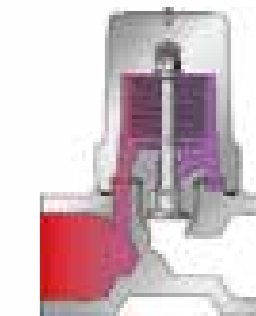
3 热冷凝水继续排放，接近饱和蒸汽温度时双金属元件关闭阀门。
