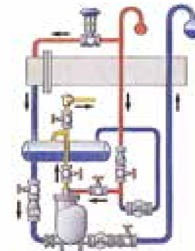
自动泵和浮球疏水阀的组合
