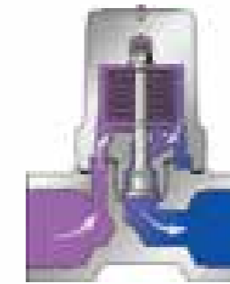
2 热的冷凝水流过疏水阀，热量使双金属元件变形，并拉动阀芯向阀座移动。
