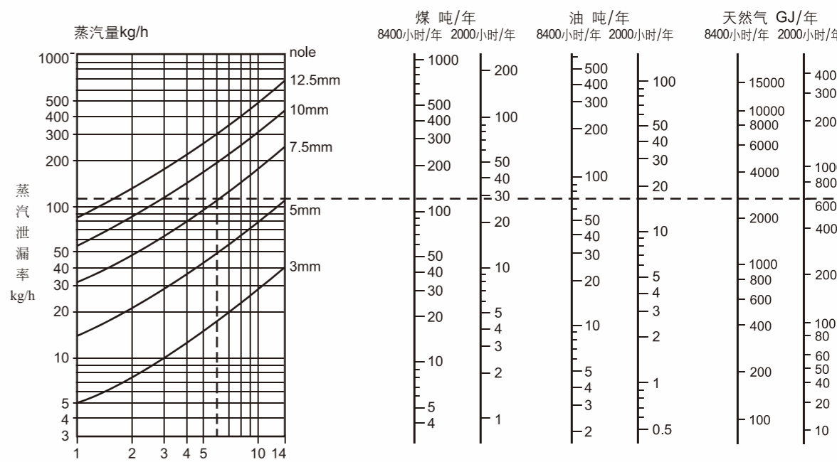
疏水阀泄漏—能量浪费示意图
