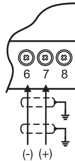
图6b. 液位变送器接线端 (自供电)
