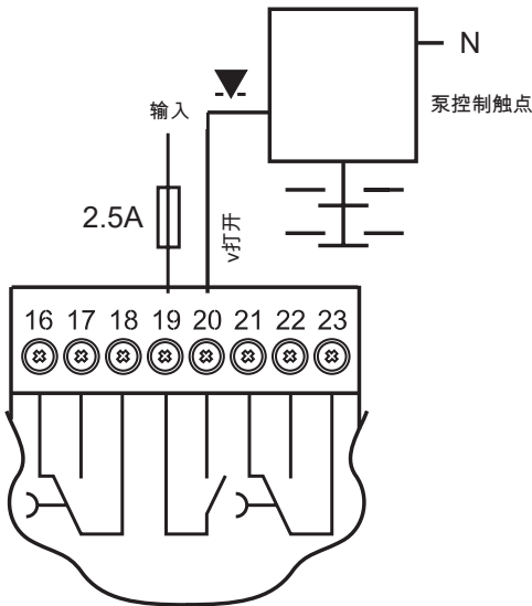
图6a. 阀门开关控制示例
