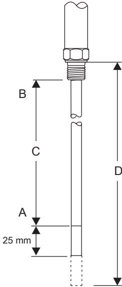
图11. 配备PA420液位变送器的LP20/21
