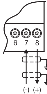
图6c. PA420液位变送器接线端 (回路供电)
