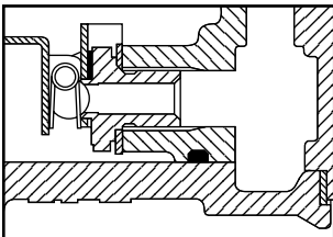
图3 DN25 (1") 主阀组件剖视图
