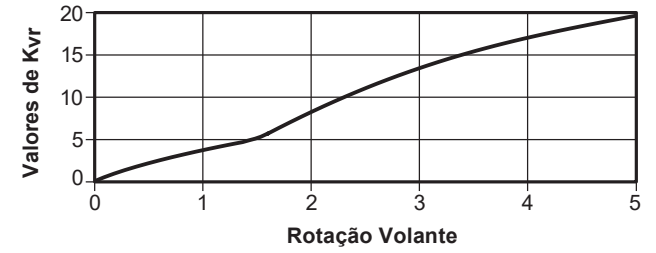
BSAT - DN32 (1 1/4")
