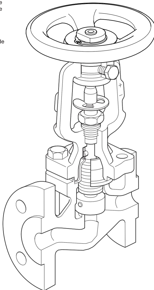
Representado BSA6T
