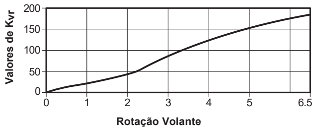
BSAT - DN100 (4")
