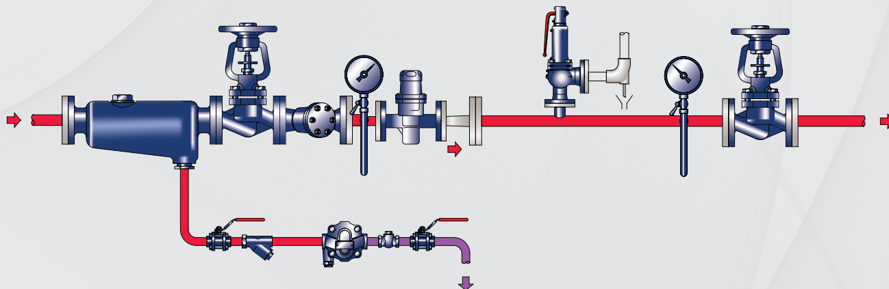
ESTAÇÃO DE VÁLVULA REDUTORA DE PRESSÃO
