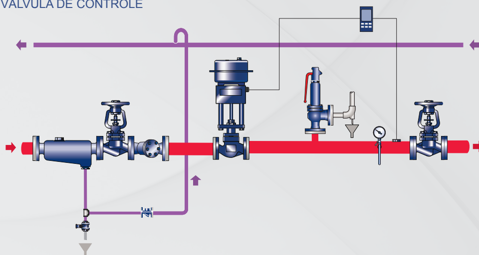
ESTAÇÃO DE VÁLVULA DE CONTROLE
