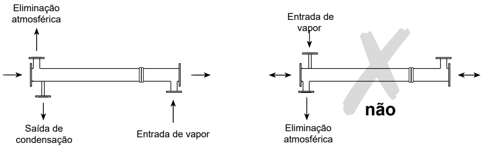
Fig. 4 e 5 - Posição quando o fluido do lado do casco está condensando vapor
