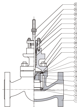
Fig. 3 - Série 85 com flanges solidários.
