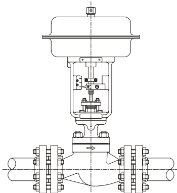
Fig. 1 - Instalação da válvula.
