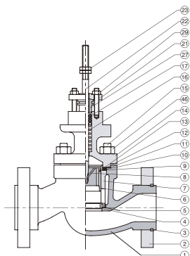
Fig. 2 - Série 85 com flanges soltos.
