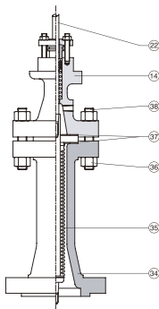
Fig. 6 - Castelo com fole de selagem.
